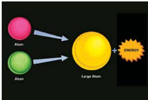
Figure 1 DEUTERIUM-DEUTERIUM FUSION
